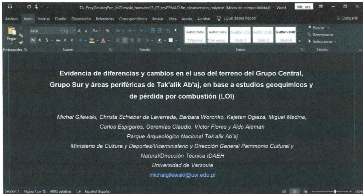
Figura 1. Captura de pantalla de la ponencia “Evidencia de diferencias y cambios en el uso del terreno del Grupo Central, Grupo Sur y áreas periféricas de Tak'alik Ab'aj, en base a estudios geoquímicos y de pérdida de combustión (LOI)” (Parque Arqueológico Nacional Tak'alik Ab'aj, MICUDE-DGPCN/IDAEH 2021).
